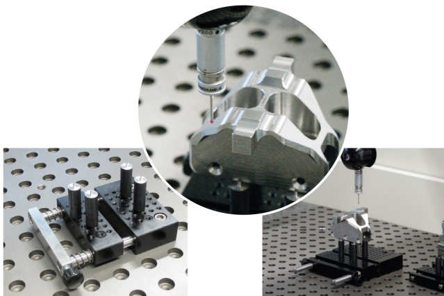
KF 50 mit speziellen Stiftbacken ausgerüstet
